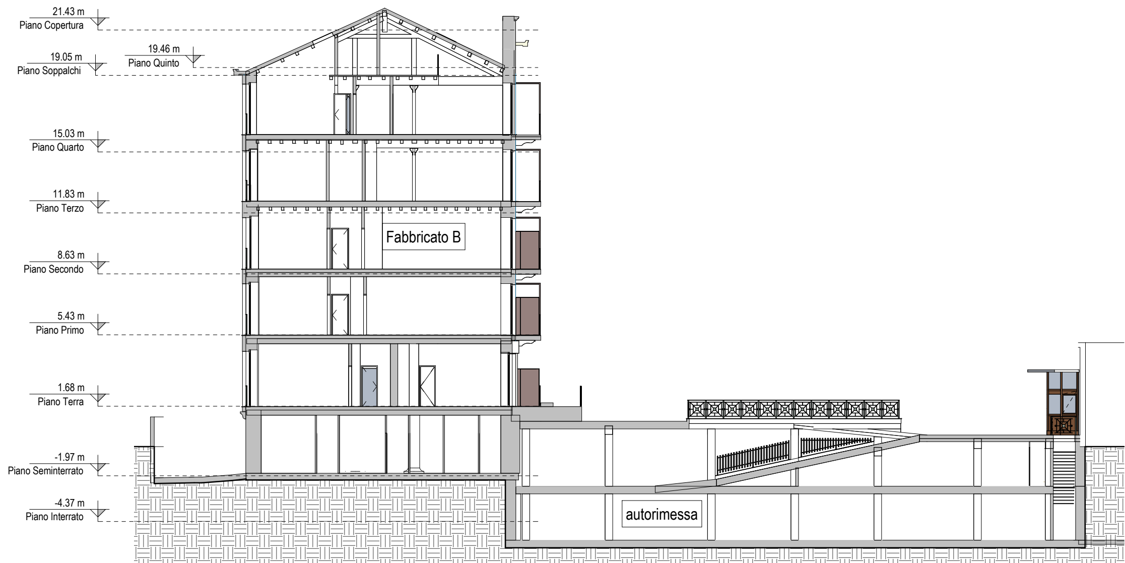
Sezione Fabbricato B
