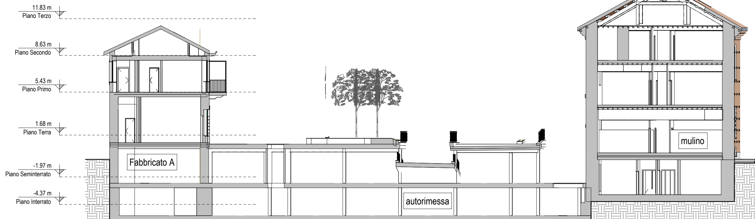
Sezione Fabbricato A
